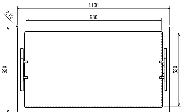
Boven aanzicht
