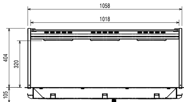
Zij aanzicht
